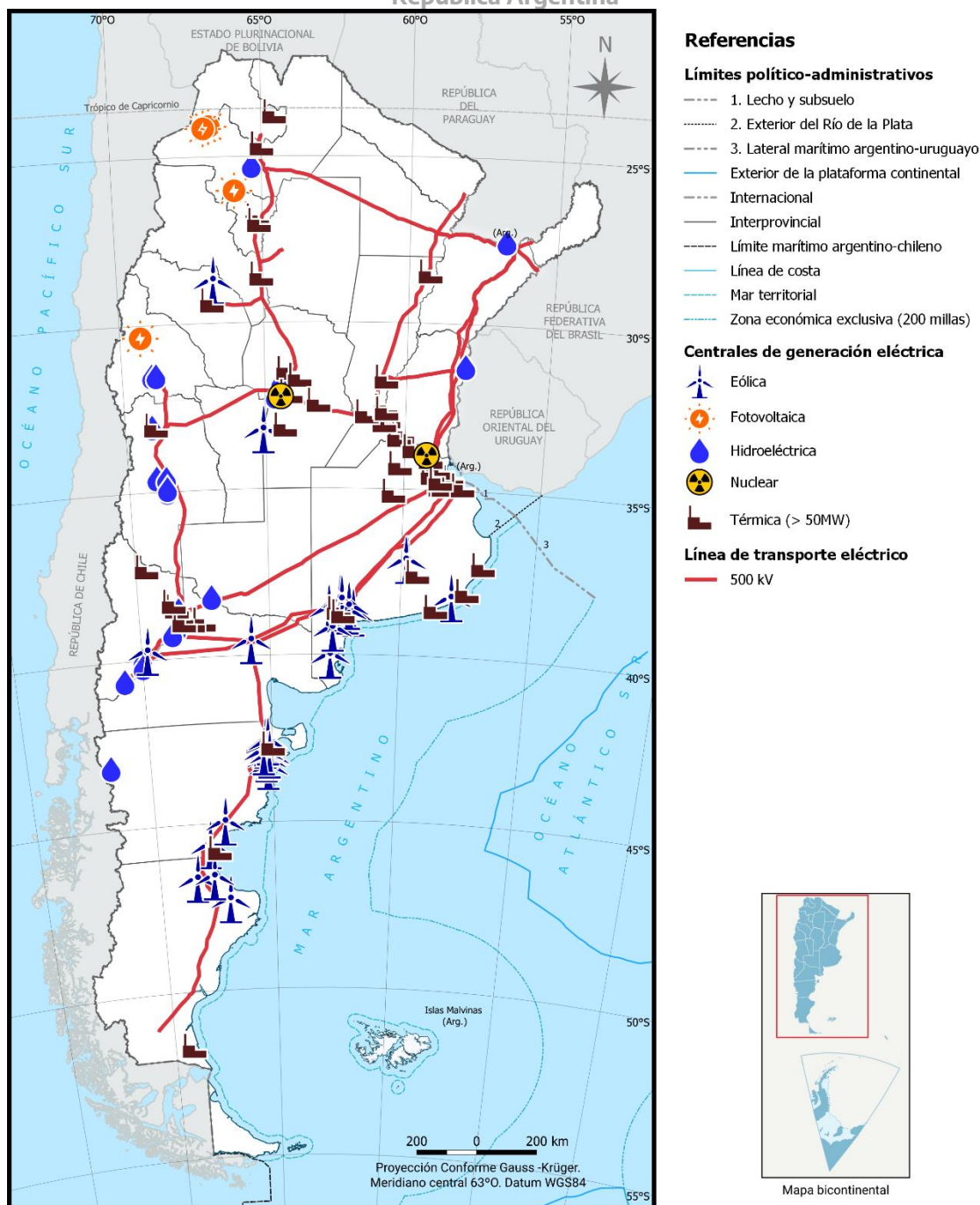
Ilustración 9: Mapa de la red eléctrica de alta tensión y centrales de generación de la República Argentina
